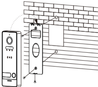
Montaż na uchwycie ściennym
