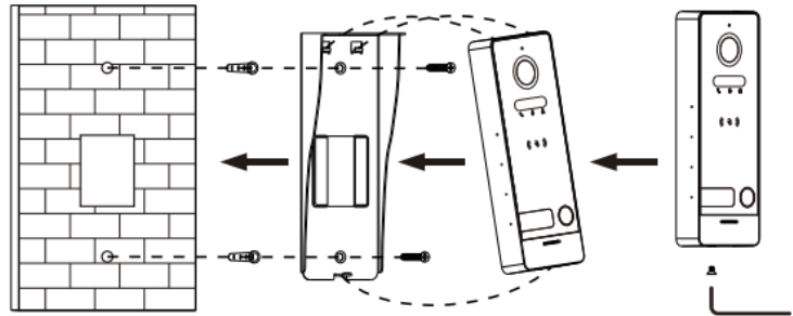
Montaż na daszku przeciwdeszczowym ( Akcesoria dodatkowe* ) *NVE-EPV100COV
