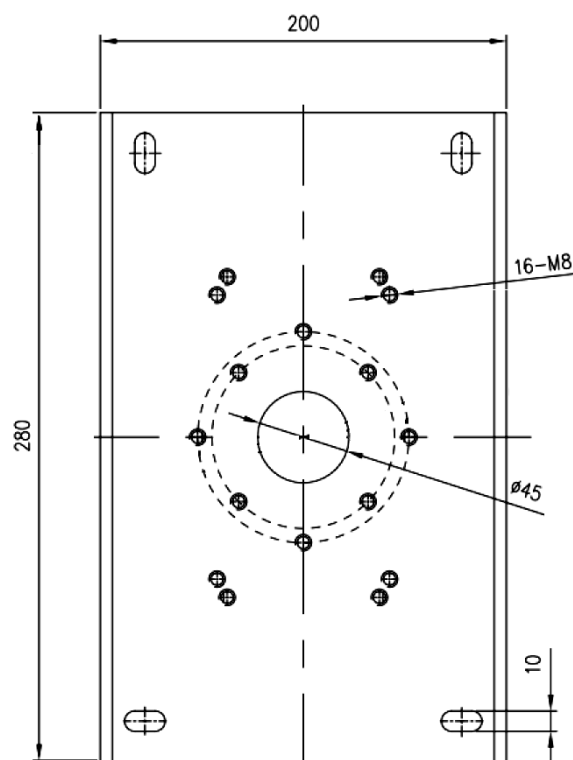
wymiary/dimensions
