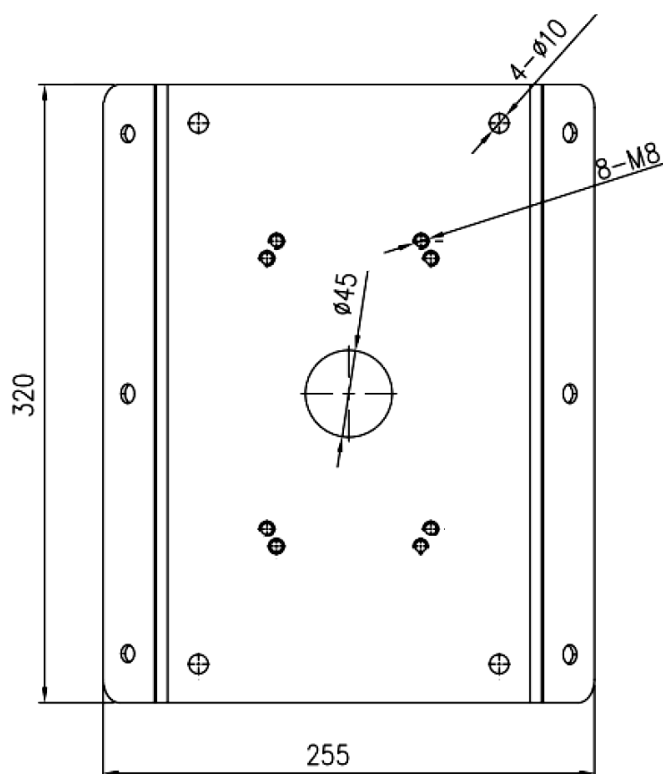
wymiary/dimensions
